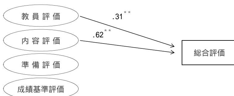
Figure 1. 授業評価因子と総合評価のパスダイアグラム
